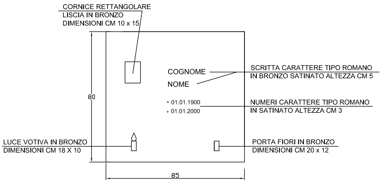
SCHEMA ACCESSORI PER LASTRA LOCULO
