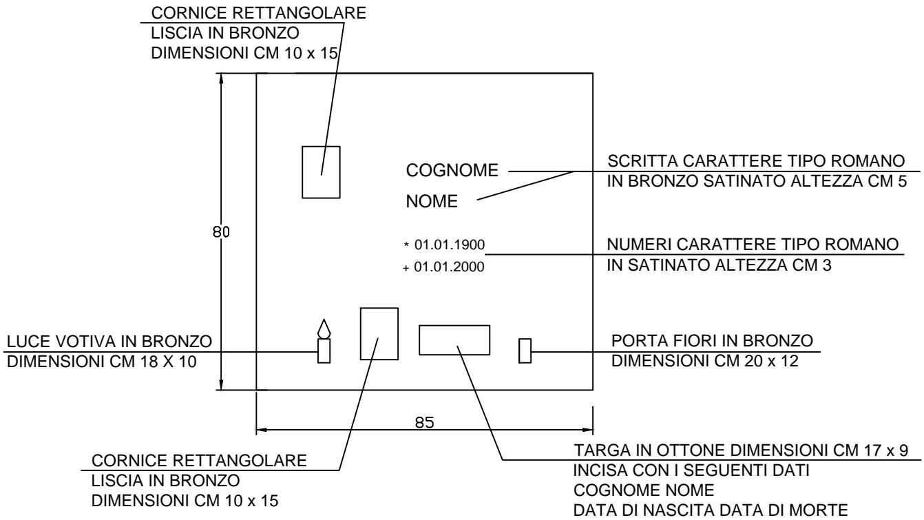
SCHEMA ACCESSORI PER LASTRA LOCULO
